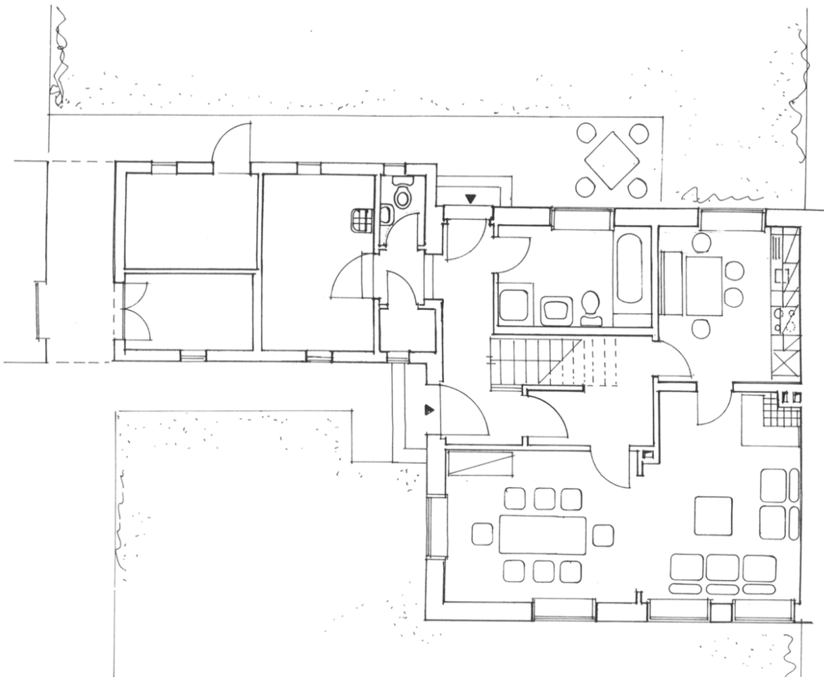
Erdgeschoß Wohnzimmer, Esszimmer, Küche, Wirtschaftsraum, Badezimmer 2, Gästetoilette, Fahrradraum
